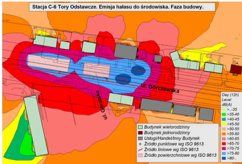
Rysunek 6. Stacja C6 torów odstawczych, emisja hałasu do środowiska w fazie realizacji, pora dzienna
