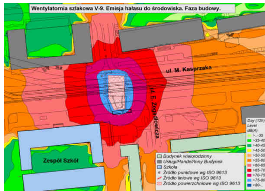
Rysunek 7. Wentylatornia V9, emisja hałasu do środowiska w fazie realizacji, pora dzienna
