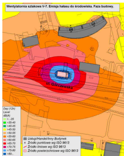
Rysunek 9. Wentylatornia V7, emisja hałasu do środowiska w fazie realizacji, pora dzienna
