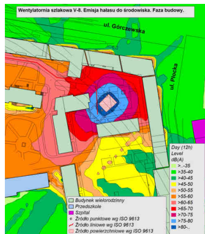
Rysunek 8. Wentylatornia V8, emisja hałasu do środowiska w fazie realizacji, pora dzienna
