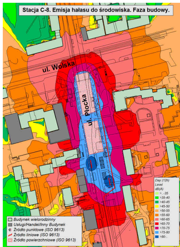
Rysunek 3. Stacja C8, emisja hałasu do środowiska w fazie realizacji, pora dzienna
