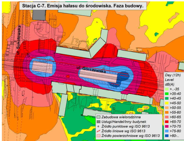
Rysunek 4. Stacja C7, emisja hałasu do środowiska w fazie realizacji, pora dzienna
