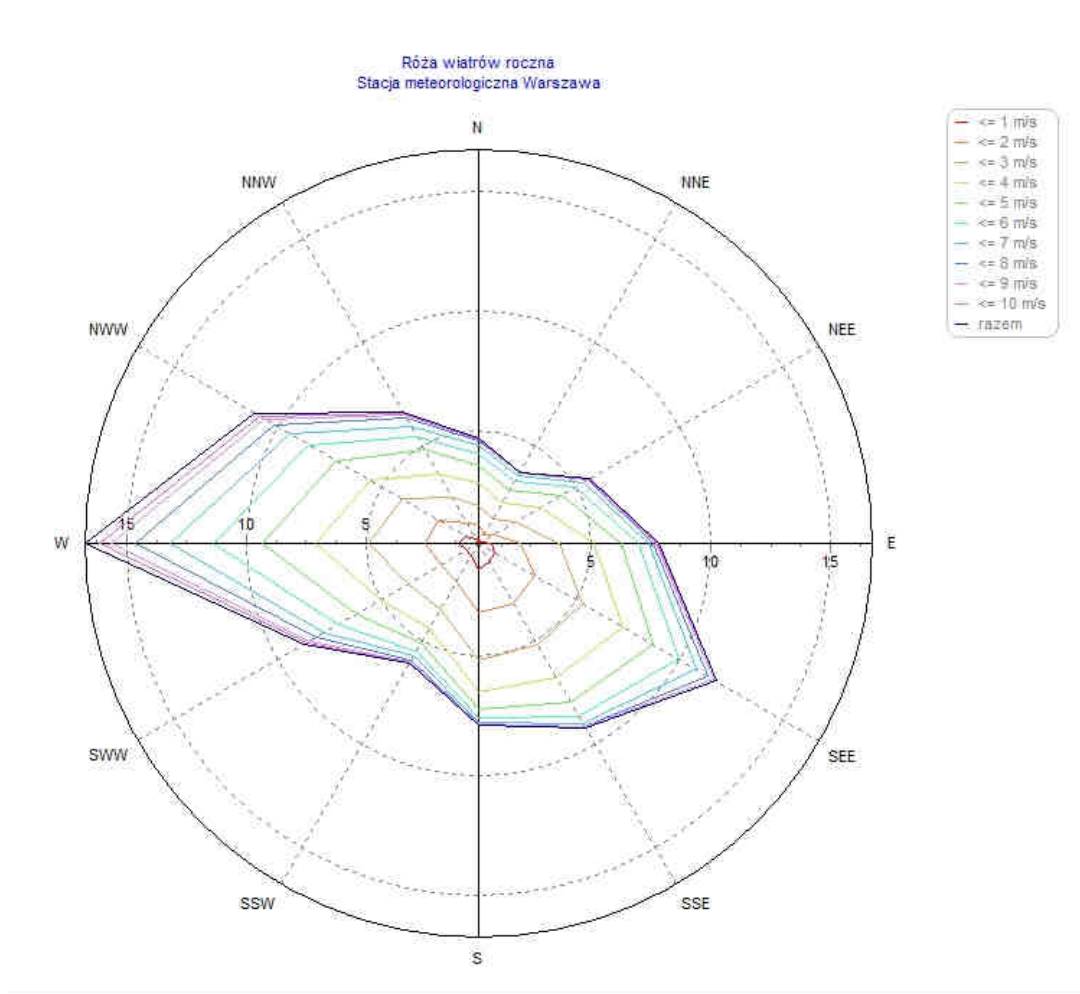
Rysunek 10. Róża wiatrów ze stacji meteorologicznej Warszawa-Okęcie
