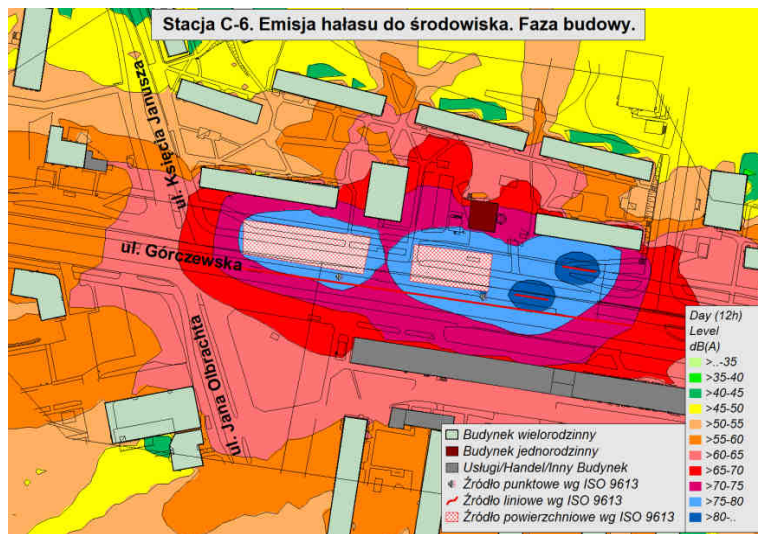
Rysunek 5. Stacja C6, emisja hałasu do środowiska w fazie realizacji, pora dzienna
