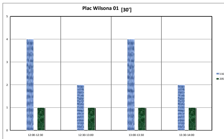
Wykres 2. Częstotliwości kursowania w godzinach 12:00 – 14:00 na przystanku Plac Wilsona 01.
