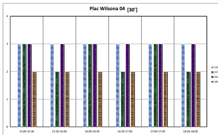
Wykres 12. Częstotliwości kursowania w godzinach 15:00 – 18:00 na przystanku Plac Wilsona 04.
