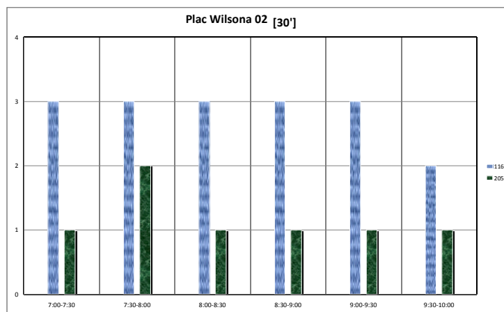
Wykres 4. Częstotliwości kursowania w godzinach 7:00 – 10:00 na przystanku Plac Wilsona 02.
