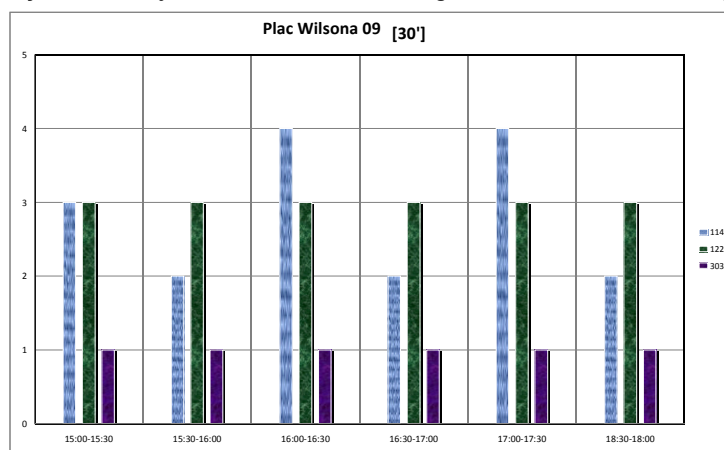
Wykres 27. Częstotliwości kursowania w godzinach 15:00 – 18:00 na przystanku Plac Wilsona 09.
