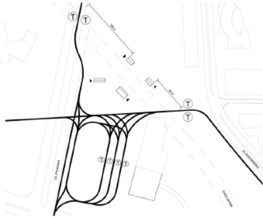
SCHEMAT PĘTLI TRAMWAJOWEJ NA KOND. 00
